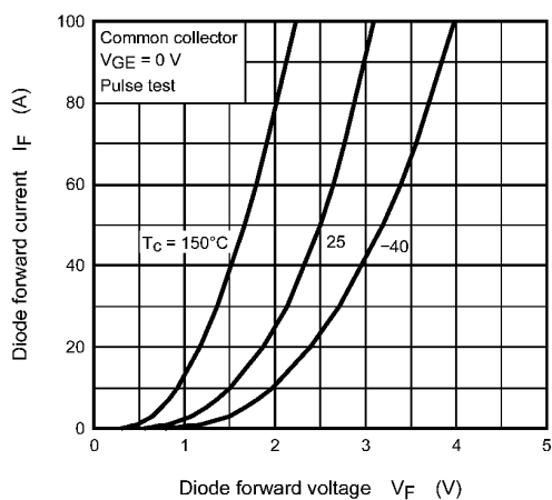
Fig. 8.17 I_F - V_F
