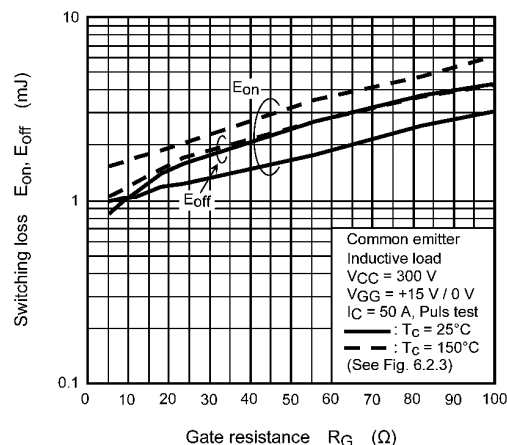
Fig. 8.14 E_{on} , E_{off} - R_G
