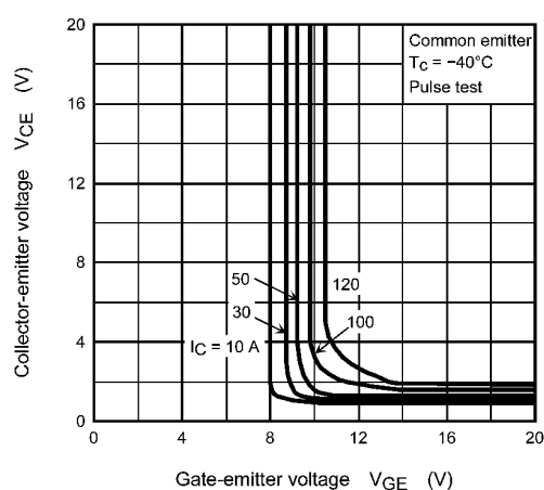
Fig. 8.6 V_{CE} - V_{GE}
