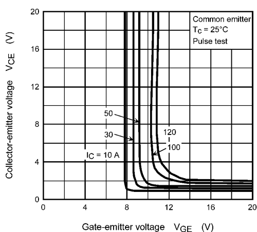
Fig. 8.5 V_{CE} - V_{GE}
