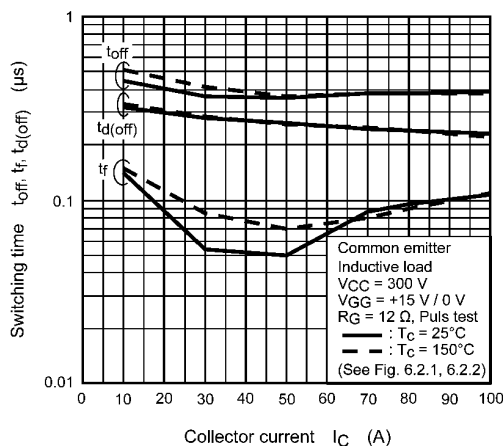
Fig. 8.13 t_{off} , t_r , t_d(off) - I_C
