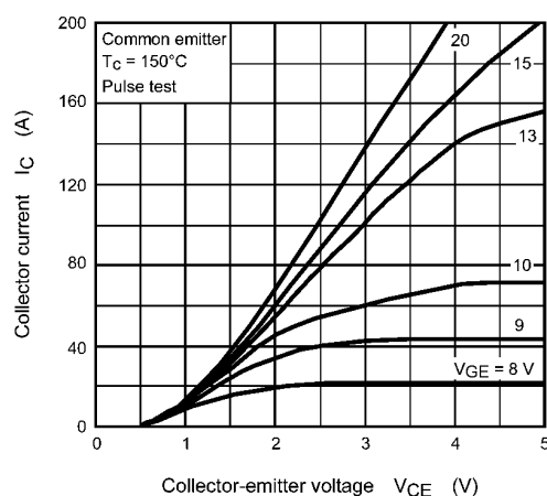
Fig. 8.4 I_C - V_{CE}
