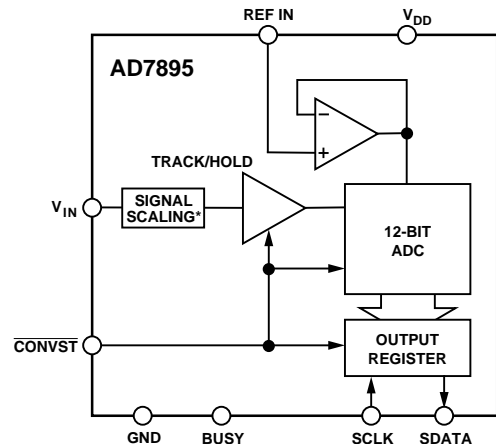
*AD7895-10, AD7895-3
