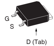
TO-252 (IXTY..HV)
