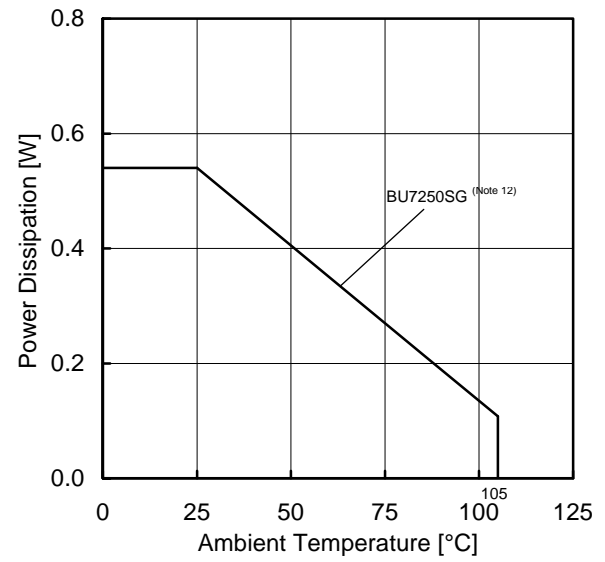
(d) BU7250SG
