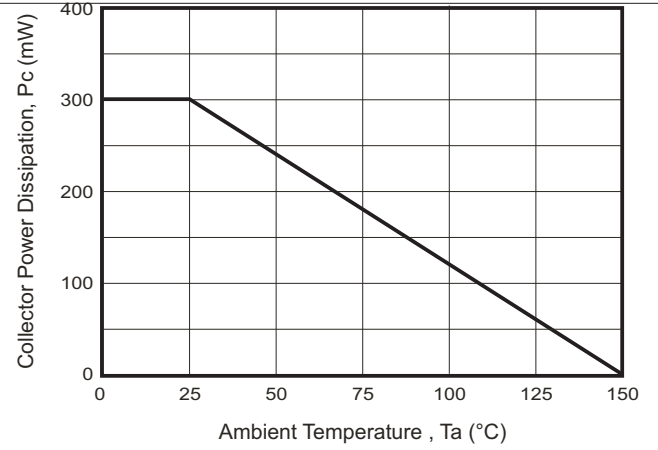
Fig. 8- P_c - T_a
