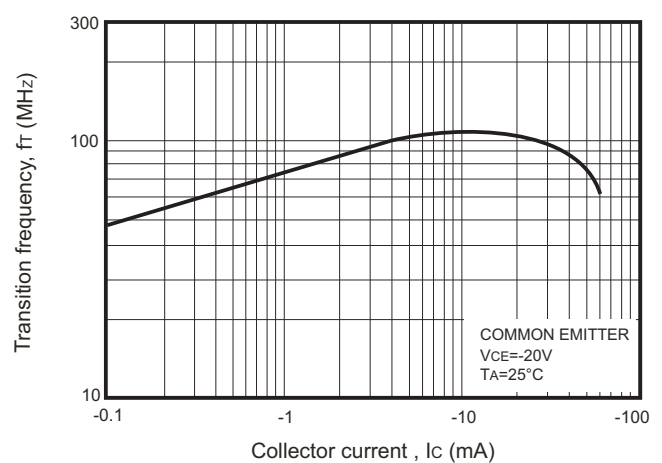
Fig.6 - f_T - I_c
