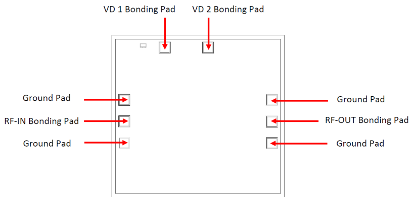
Fig 2. Die Layout
