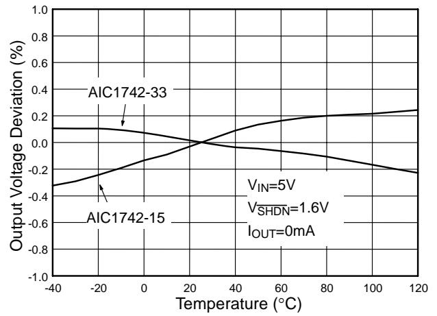
Fig. 4 Output Voltage
