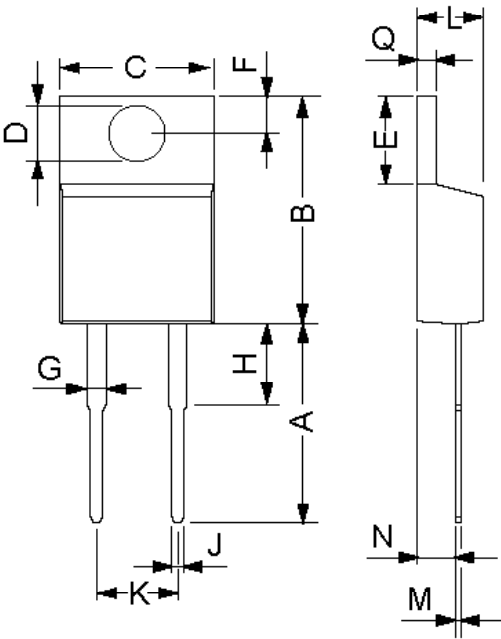
Dimensions TO-220AC
