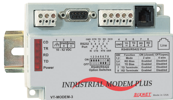
VT-MODEM -3
