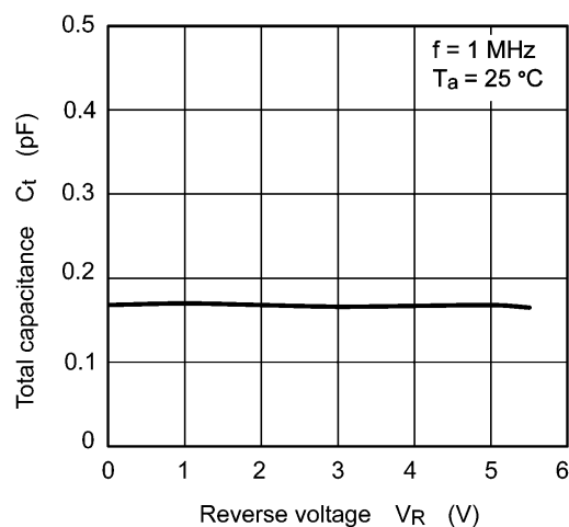
Fig. 7.3 C_t - V_R
