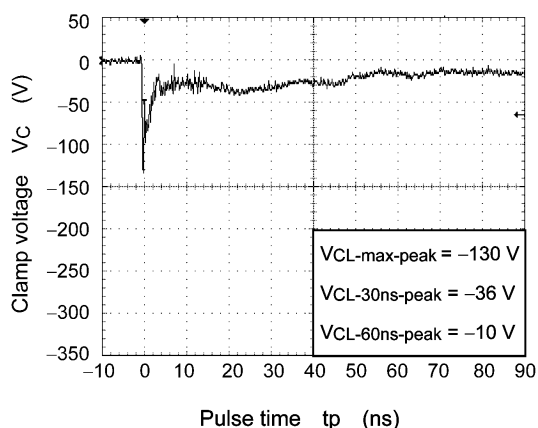
Fig. 10.4 -15 kV
