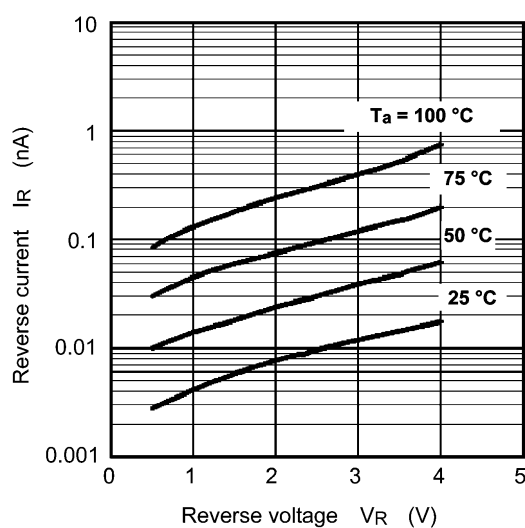
Fig. 7.2 I_R - V_R
