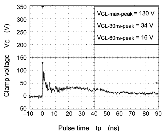
Fig. 10.3 +15 kV
