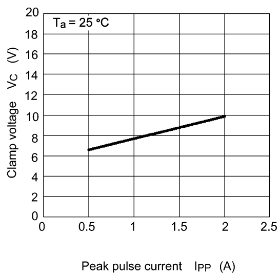
Fig. 8.1 V_C - I_{PP}
