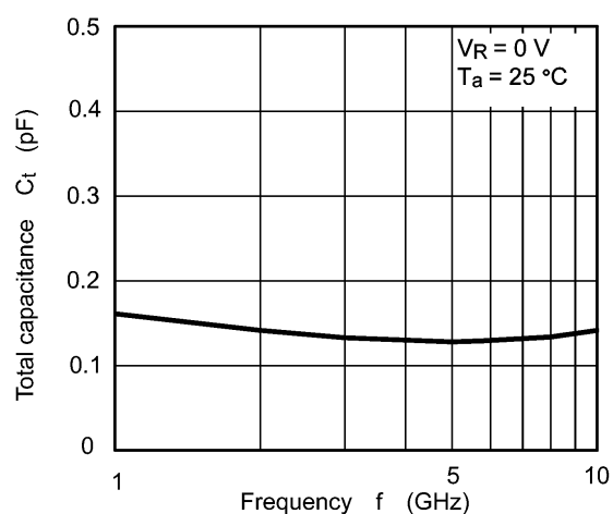
Fig. 7.4 C_t - f
