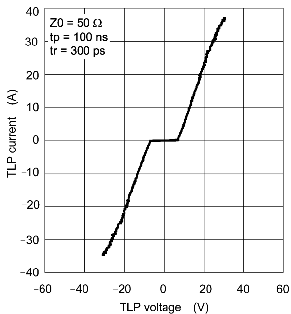
Fig. 8.3 TLP
