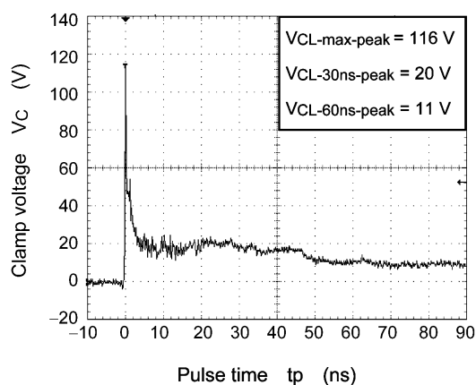
Fig. 10.1 +8 kV
