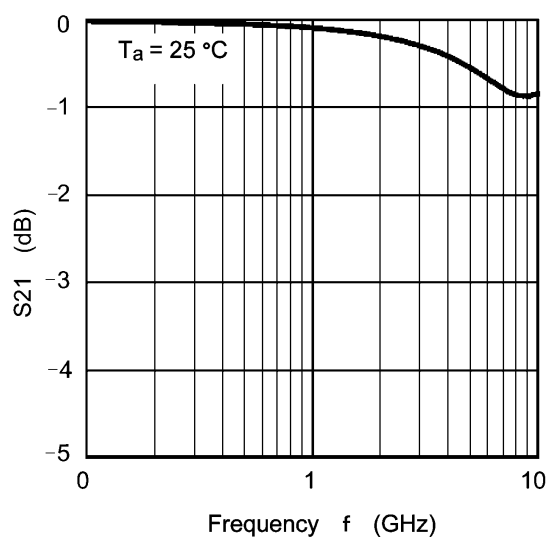
Fig. 9.1 S21 - f
