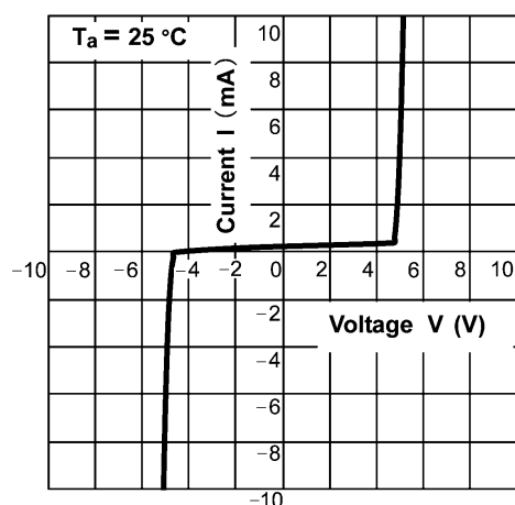
Fig. 7.1 I - V
