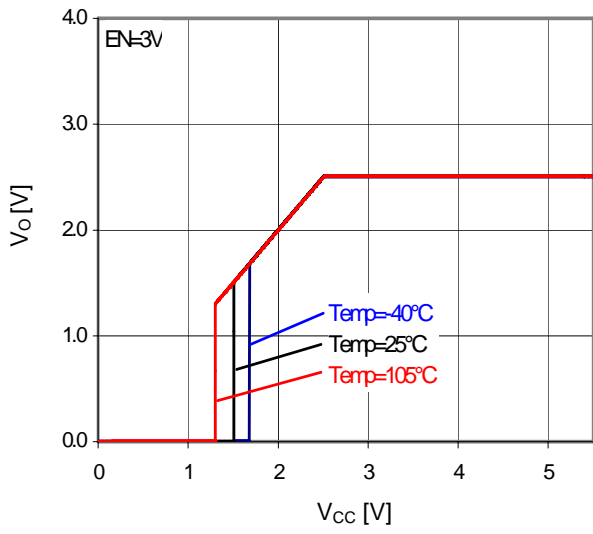
Fig.27 V_{CC}-V_o (I_o=0\text{mA})
