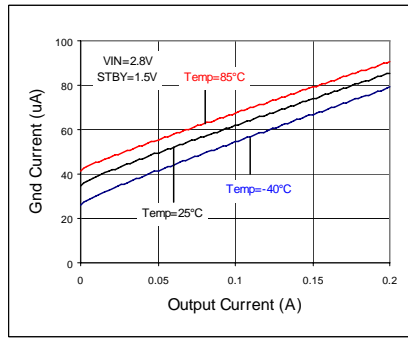
Fig 7. IOUT - IGDND
