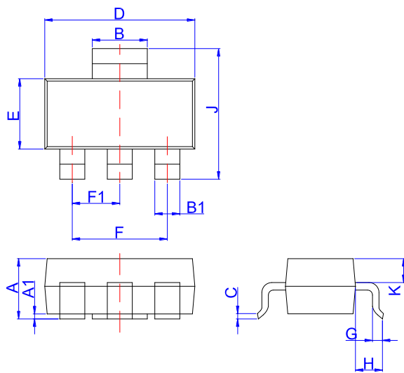
SOT-223
