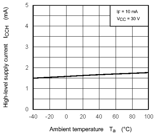
Fig. 12.2.6 I_{cCH} - T_a
