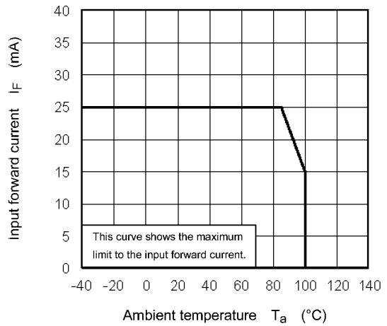
Fig. 12.2.2 I_F - T_a
