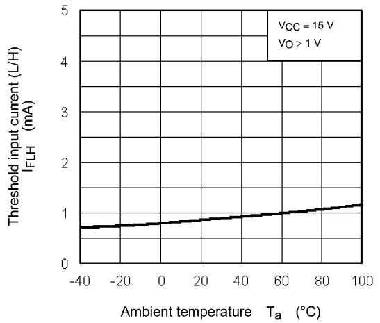
Fig. 12.2.4 I_{FLH} - T_a
