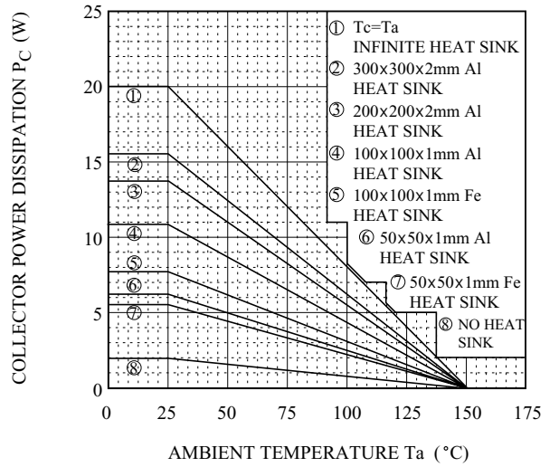
P_c - T_a
