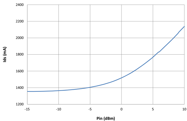
I ds versus Pin (Vd=5V)
