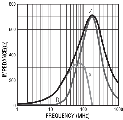
MH 1608- 601Y
