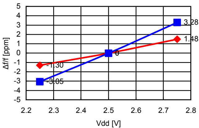
fcenter=20MHz, Vdd=2.5V±10%
