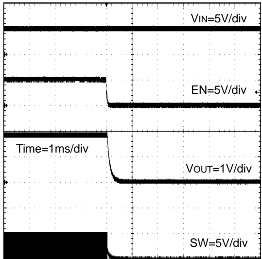
Figure 29. Power Down (EN = 5V to 0V)
