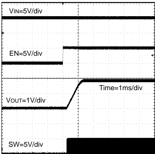
Figure 28. Power Up (EN = 0V to 5V)
