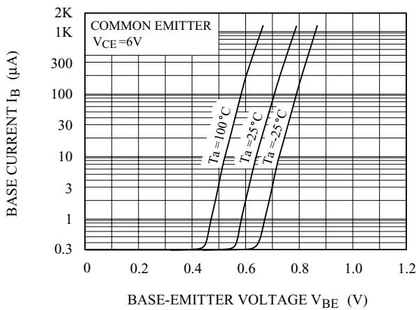
I_B - V_{BE}
