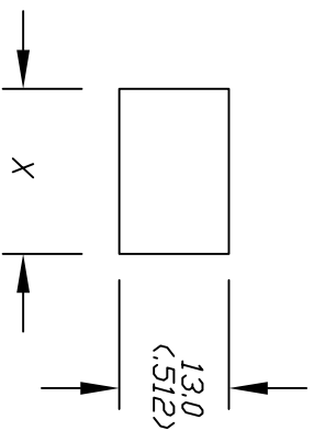
RECOMMEND P.C.B. LAYOUT
