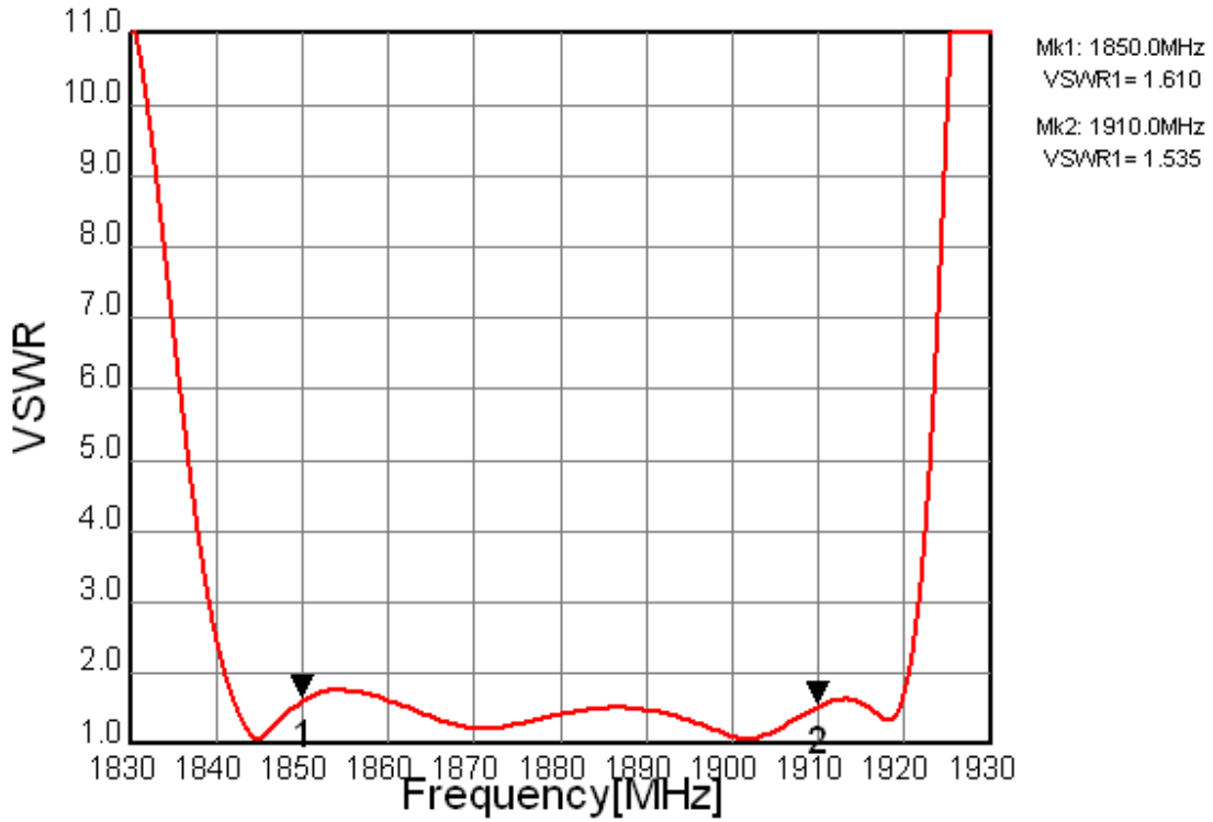
Fig.4 Input VSWR
