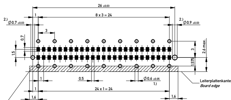
Leiterplatten-Layout Vorschlag / PCB-Layout Proposal
