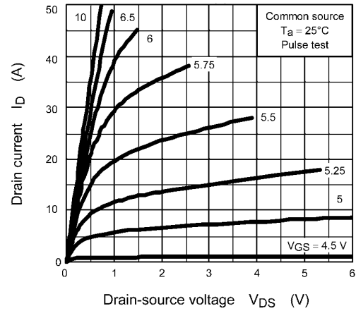
Fig. 8.2 I_D - V_{DS}
