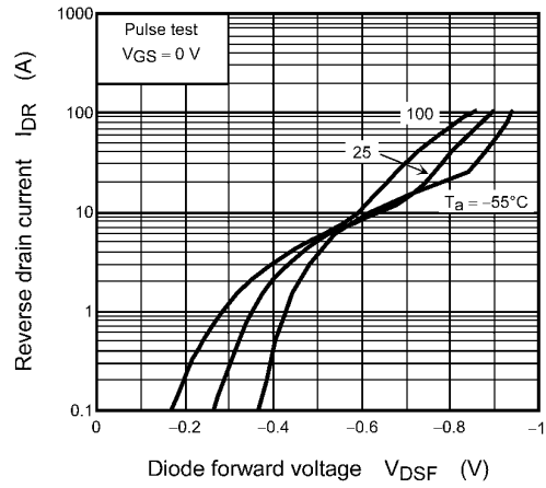
Fig. 8.15 I_{DR} - V_{DSF}
