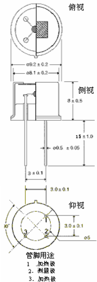
结构及尺寸
