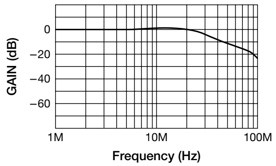
■ Vout
