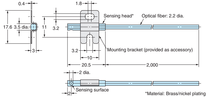
E32-M21
