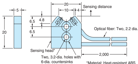
E32-L25
