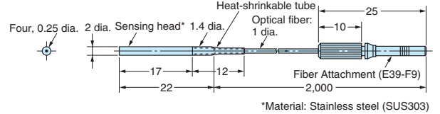
E32-T22B
