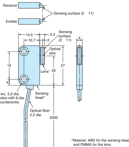
E32-T16J E32-T16JR
