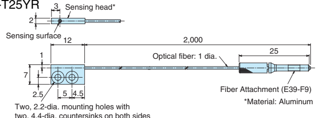
E32-T25Y E32-T25YR
