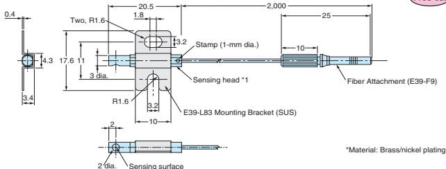
E32-A03
