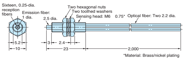
E32-CC200 E32-CC200R
