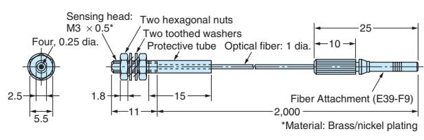
E32-T221B
