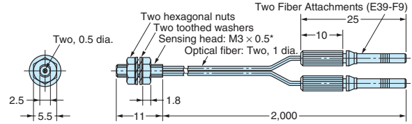
E32-DC200E E32-D21R
