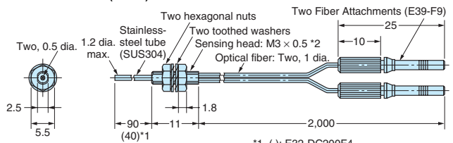
E32-DC200F(F4) E32-DC200FR(F4R)
