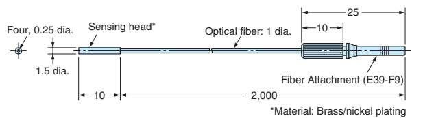
E32-T25XB
