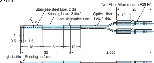
E32-D24 E32-D24R
