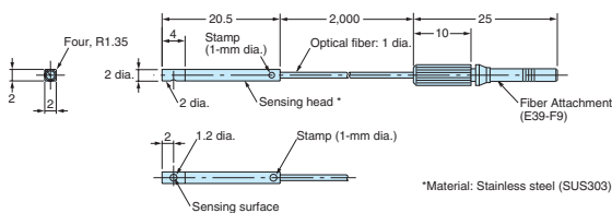
E32-A04
