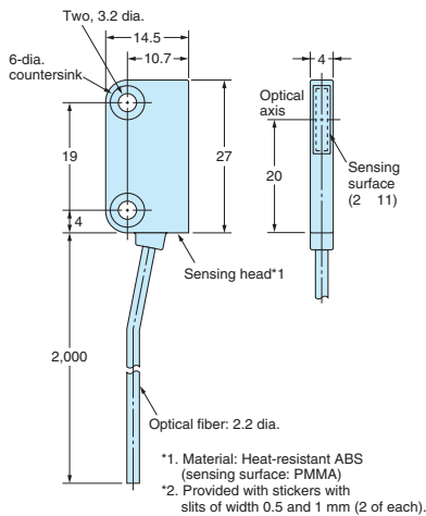
E32-T51
