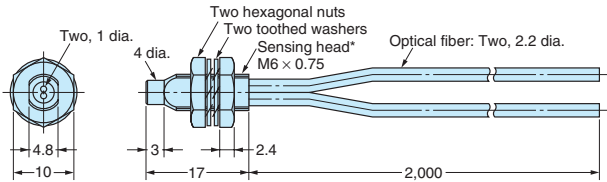
E32-DC200 E32-D11R
