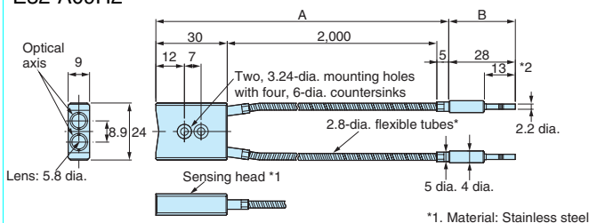
E32-A09H2
