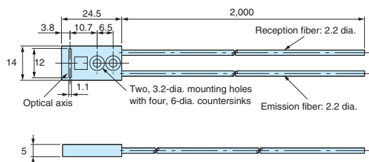
E32-A08 E32-A07E1(E2)
