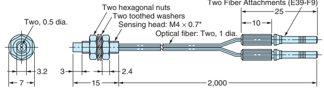
E32-DC200E E32-D21R
