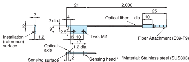
E32-A04-1
