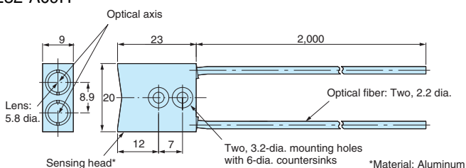
E32-A09 E32-A09H
