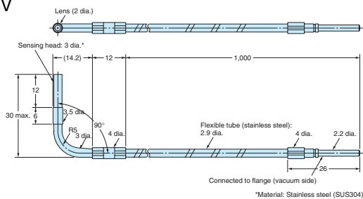
E39-F1V
