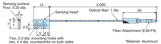
E32-T25XB
