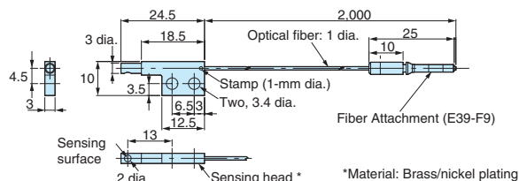
E32-A03-1
