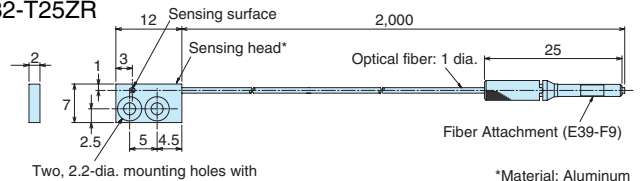
E32-T25Z E32-T25ZR
