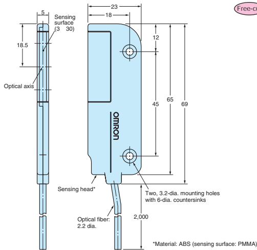
E32-T16J E32-T16JR
