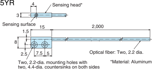
E32-T15Y E32-T15YR
