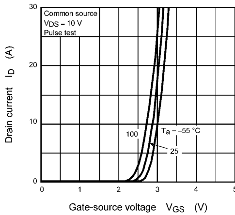
Fig. 8.3 I_D - V_{GS}
