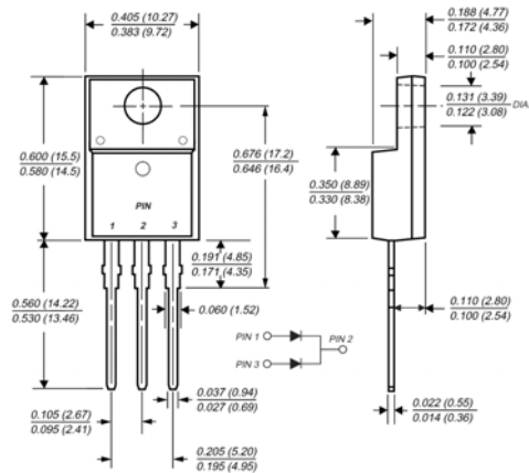
ITO-220AB
