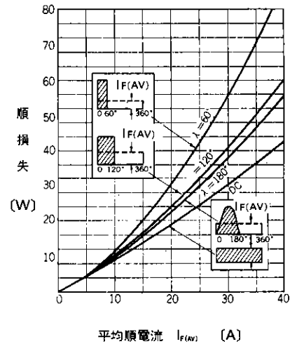
平均順電流 I_{F(AV)} (A) 順損失
