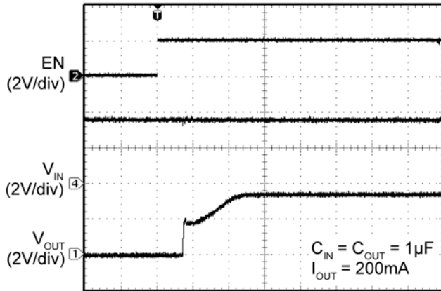
Enable Turn-On
