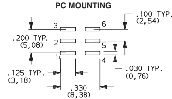
GT22-omit pads 2 & 5.
