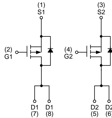
P-Channel MOSFET
