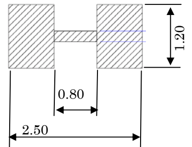
・内部電極形状
