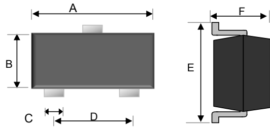
SOT-323
