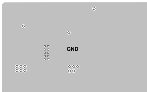
Inner Layer 1
