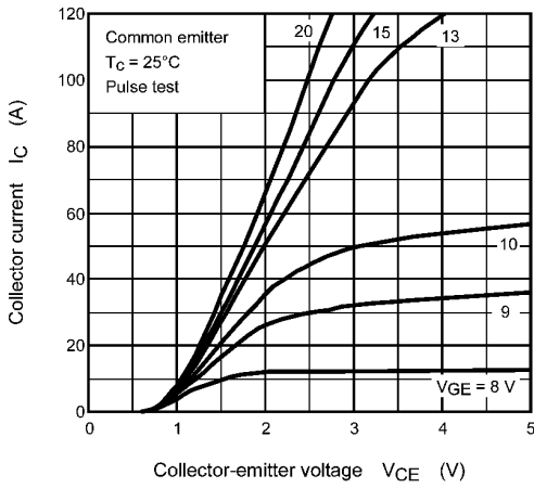
Fig. 8.1 I_c - V_{ce}
