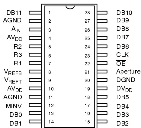
28 Pin SOP (EIAJ, 8.4mm)
