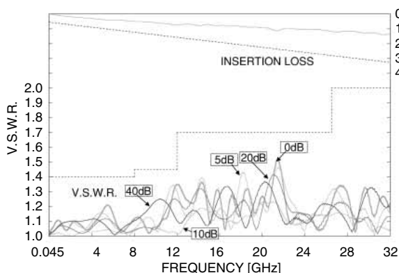
P-AT-9(32-75)A(40)
