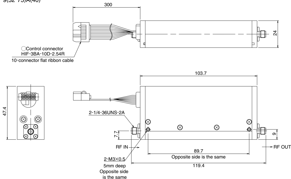
P-AT-9(32-75)A(40)
