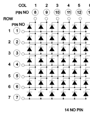
BL-M13A671
