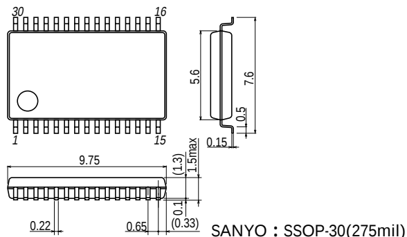
外形図 3191A (unit : mm)
