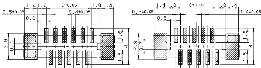
基板取付法 (奇数ピン)
