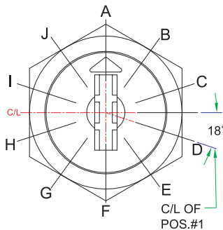
36° INDEXING
