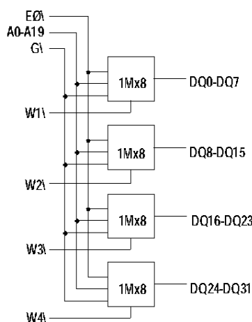
EDI7F341MV-BNC 1Megx32 80 pin SIMM
