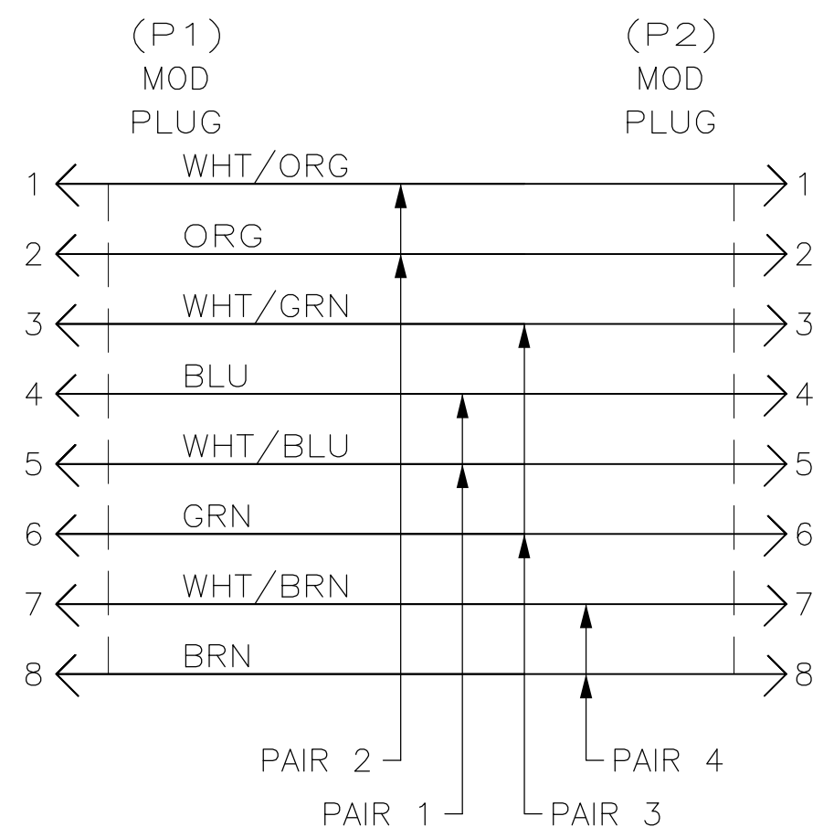
WIRING DIAGRAM 568B
