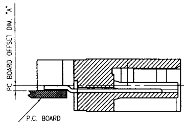
SEC. A-A
