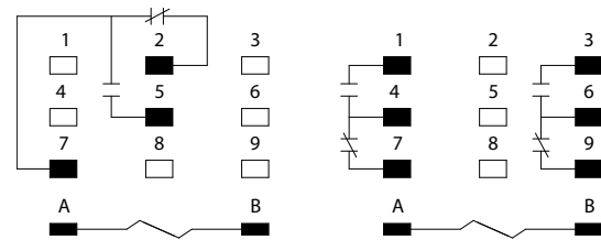
SPDT
