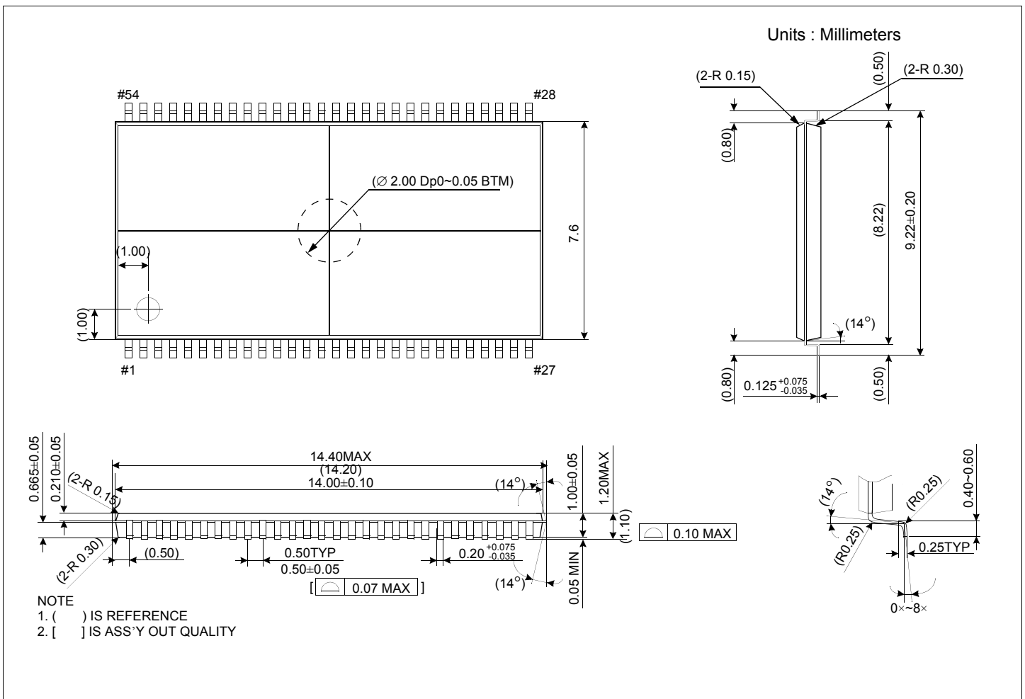
54pin sTSOP II-300 / Package dimension
