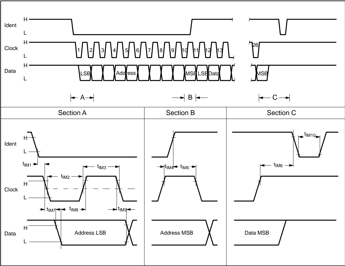
Fig. 2-16: IM Bus waveforms
